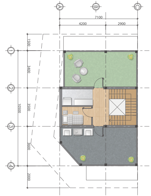
MB TẦNG THƯỢNG - 1/100
