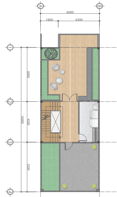
MB TẦNG THƯỢNG - 1/100
