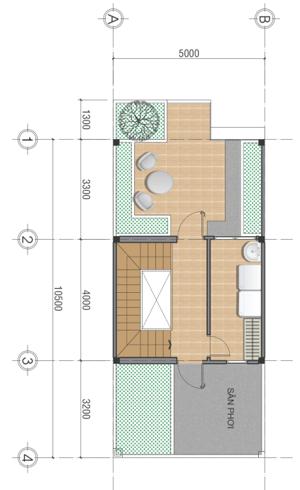
MB TẦNG THƯỢNG - 1/100
