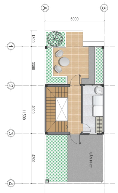
MB TẦNG THƯỢNG - 1/100
