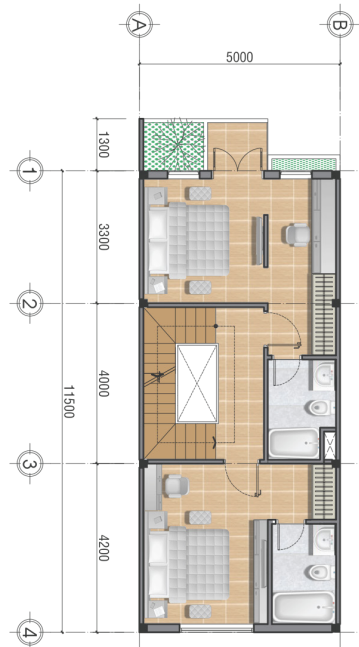
MB TẦNG 2,3 - 1/100
